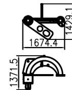
注浆弯头 870kg
