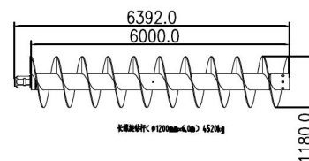
长螺旋钻杆 4520kg CFA Drill Rod
