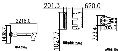
刮土器590kg 吊锚架楔块258kg 主滑轮架50kg Frame Wedge Block 258kg Main Pulley Frame 50kg
