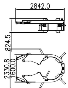
导向架 (1270) kg Guide Frame (1270)kg
