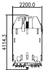
Φ3000双底双开门 截齿捞砂斗 90000kg Φ3000 Double- Bottom, Double- Door Cutterhead
